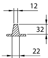
Querschnitt A-A
