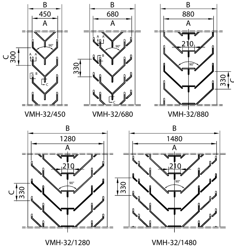
Profilausführung B-B
