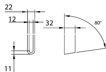
Profilausführung C-C
