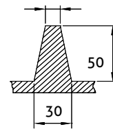
Querschnitt A-A
