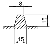
Querschnitt A-A
