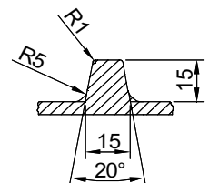
Profilausführung B-B
