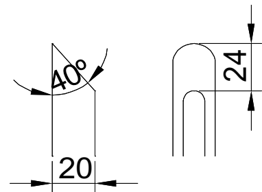
Profilausführung B-B
