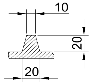
Querschnitt A-A
